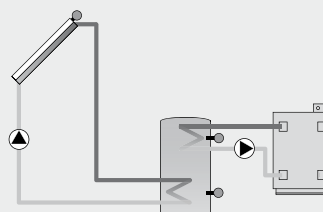
Esempio 03: Sistema solare con 1 accumulatore e riscaldamento integrativo
