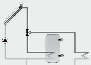
Esempio 10: Sistema solare con 1 accumulatore e deviazione calore in eccesso
