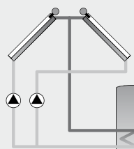
Esempio 07: Sistema solare con tetto rivolto a est/ovest
